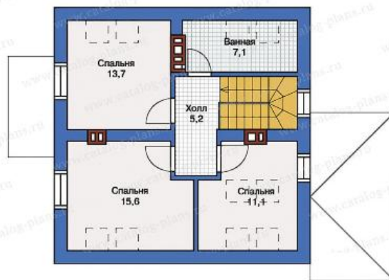
План второго этажа
